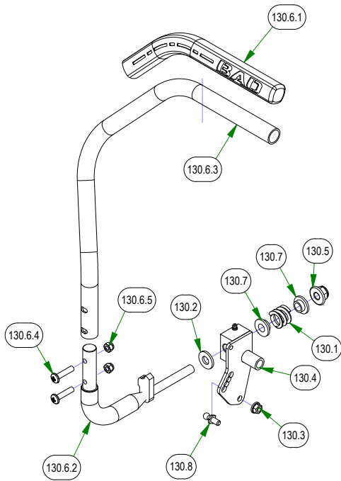
031-0018-23 ZT Steering Arm Assembly-Right Hand
